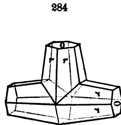
Pyrrhotite.
